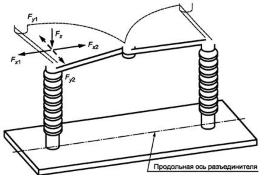
Рисунок 1 - Пример приложения механических нагрузок к выводам двухколонкового разъединителя
